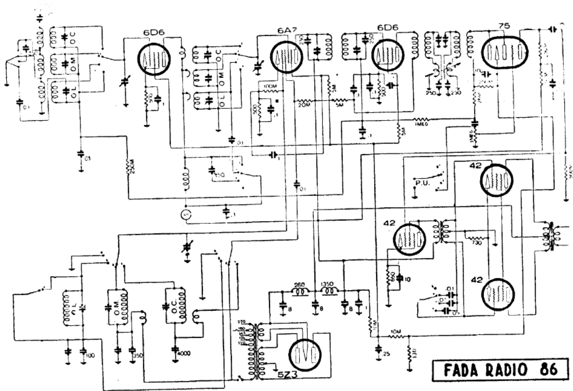
FADA RADIO. - La Precisa. - Mod. « 86 ». - Produzione 1937. - Media frequenza: 470 kHz.
